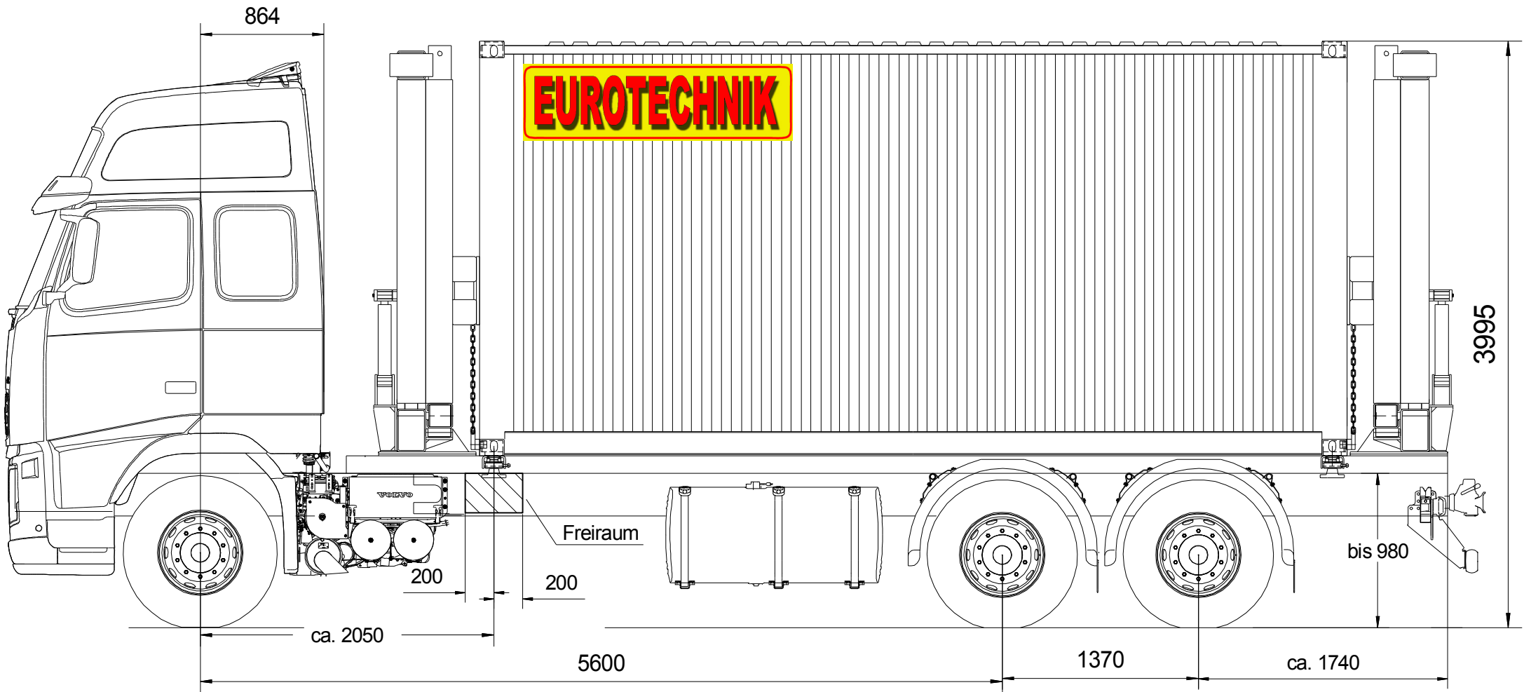
VOLVO FH12 26 to Radstand 5600+1370mm. ET-SLV Seitenlader Vertikal
