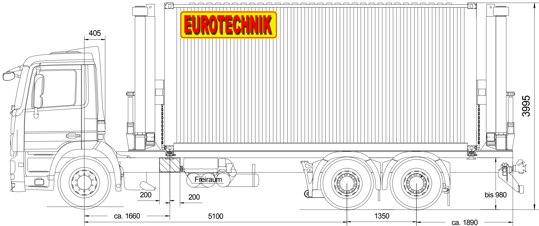
MB ACTROS 25 to Radstand 5100+1350mm. ET-SLV Seitenlader Vertikal
